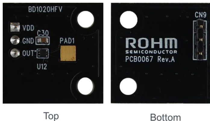
Figure 7. 基板の写真
