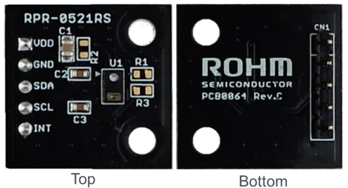
Figure 7. 基板の写真
