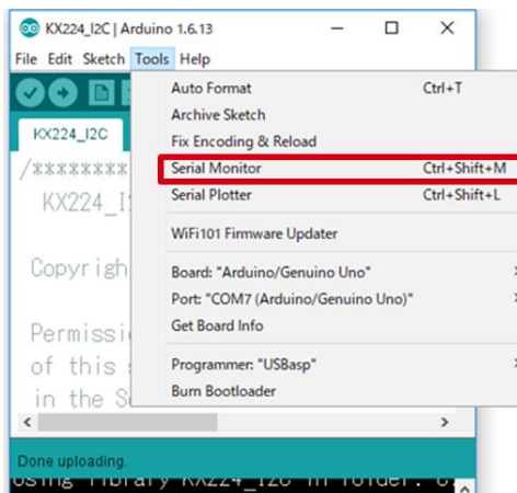
Figure 5. Tools 設定
