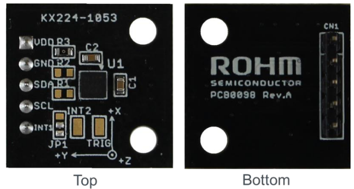
Figure 7. 基板の写真
