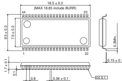
SSOP-A44
