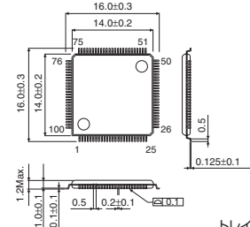
TQFP100V
