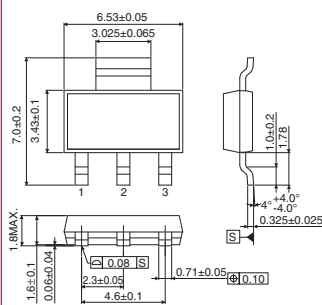
SOT223-4
