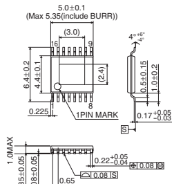
HTSSOP-B16
