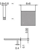
UCSP50L
