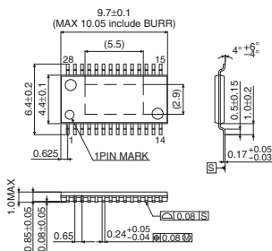
HTSSOP-B28
