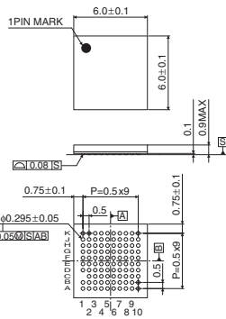
VBGA099W060
