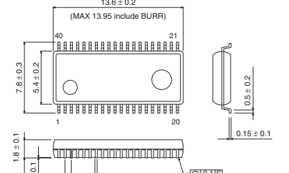
SSOP-B40
