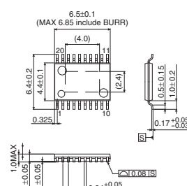
HTSSOP-B20
