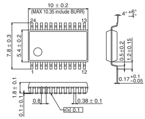
SSOP-A24
