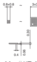
UCSP30L
