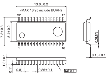
SSOP-A32
