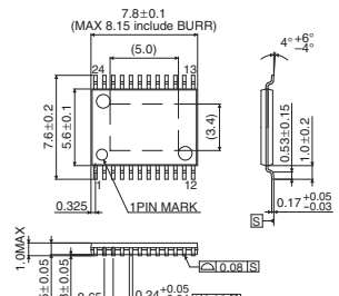
HTSSOP-B24
