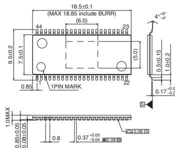
HTSSOP-A44
