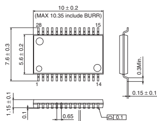
SSOP-B28
