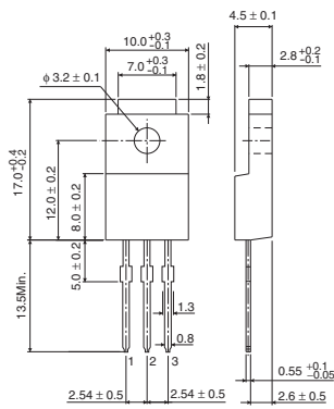
TO220FP-3
