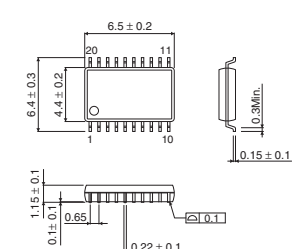
SSOP-B20
