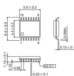
SSOP-B16
