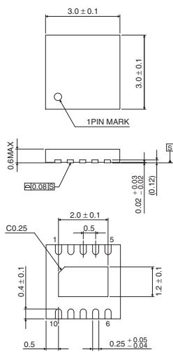
VSON010X3030
