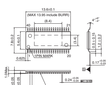
HTSSOP-B40
