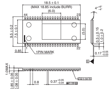
HTSSOP-A44R
