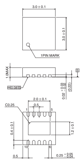
VSON010V3030
