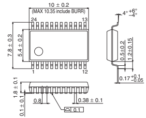
SSOP-A24
