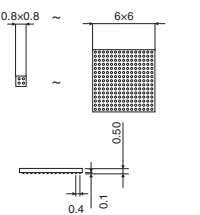
UCSP50L
