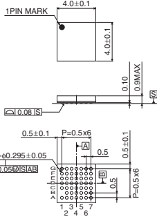
VBGA048W040
