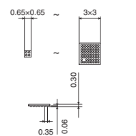
XCSP30L
