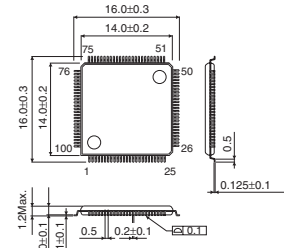
TQFP100V
