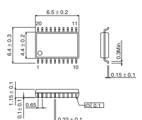
SSOP-B20
