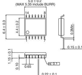
SSOP-B14
