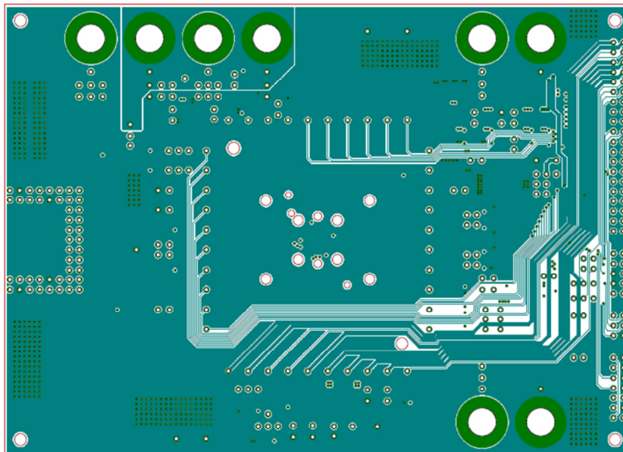
図 7. Second Layer Layout
