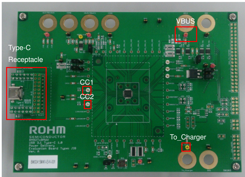
図 3. 評価ボード写真
