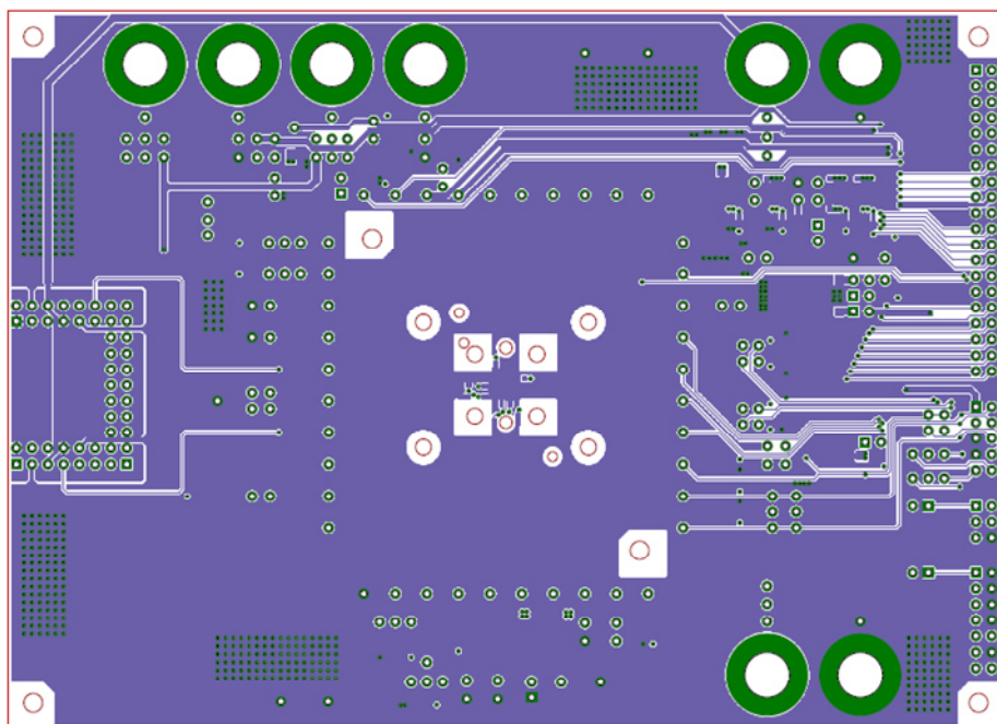
图 9. Bottom Layer Layout
