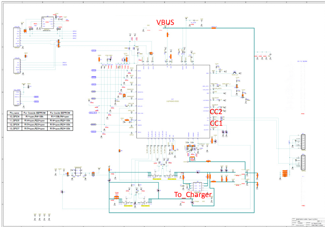
図 2. 評価ボード回路図
