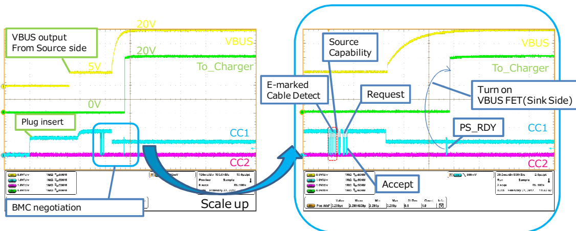
図 5. Power Delivery ネゴシエーション波形
