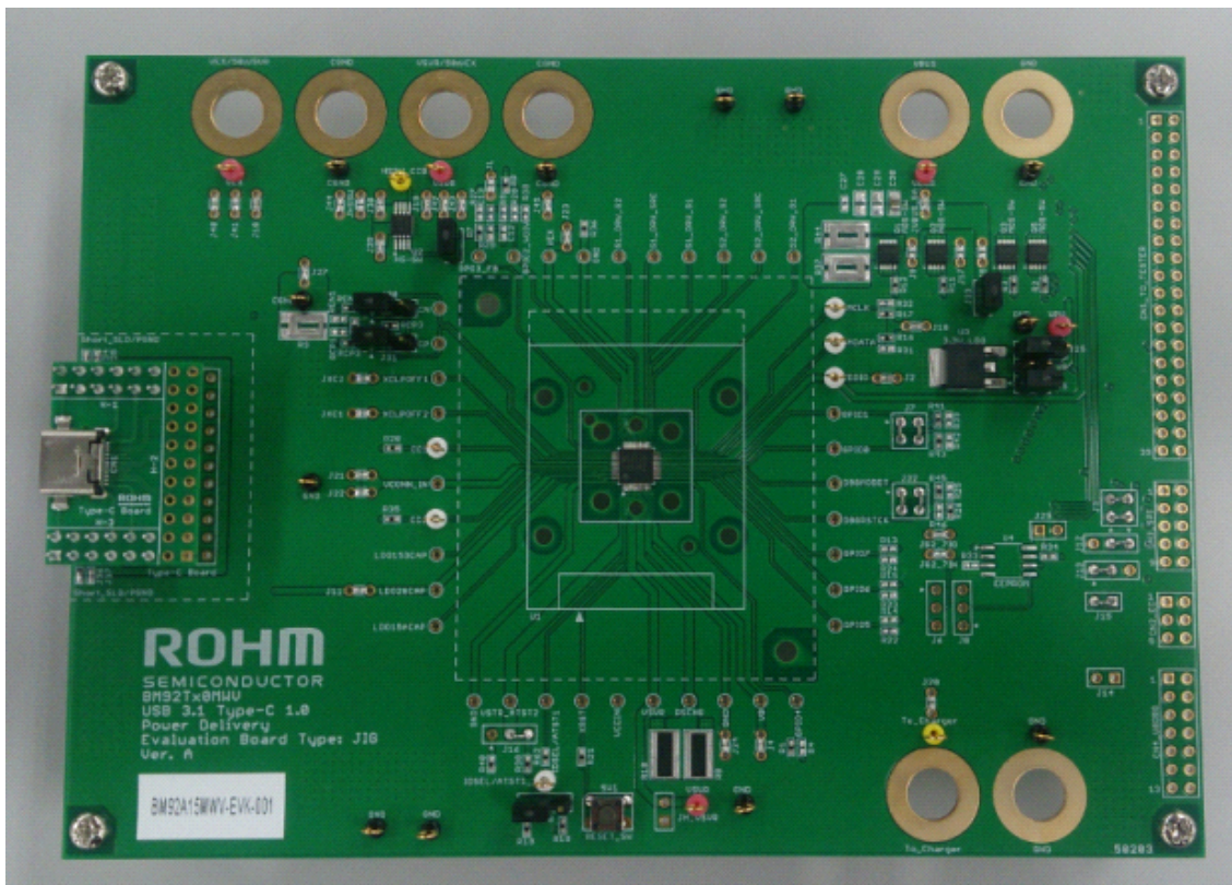
図 1. 評価ボード写真
