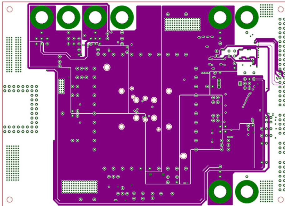
图 8. Third Layer Layout
