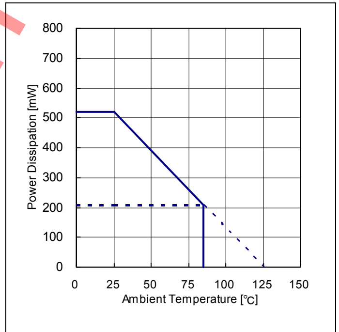
Figure 8. パッケージ熱軽減特性
