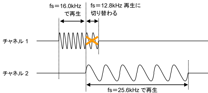
図 1) チャンネル 1 再生中にチャンネル 2 に違うサンプリング周波数を再生させた場合
