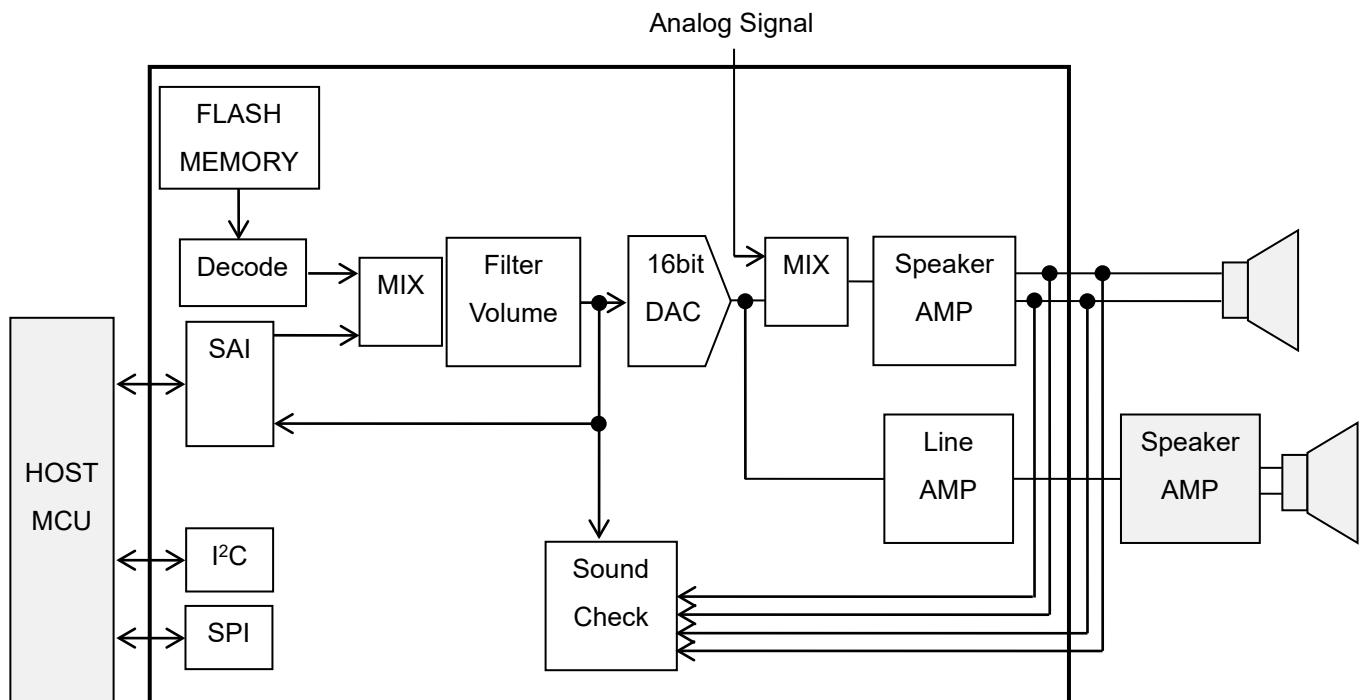
基本アプリケーション回路
