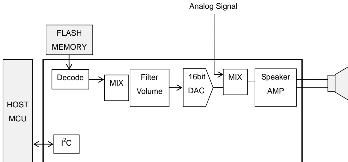
基本アプリケーション回路
