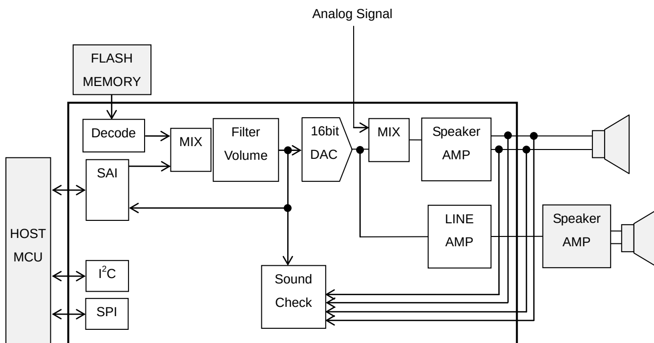
基本アプリケーション回路
