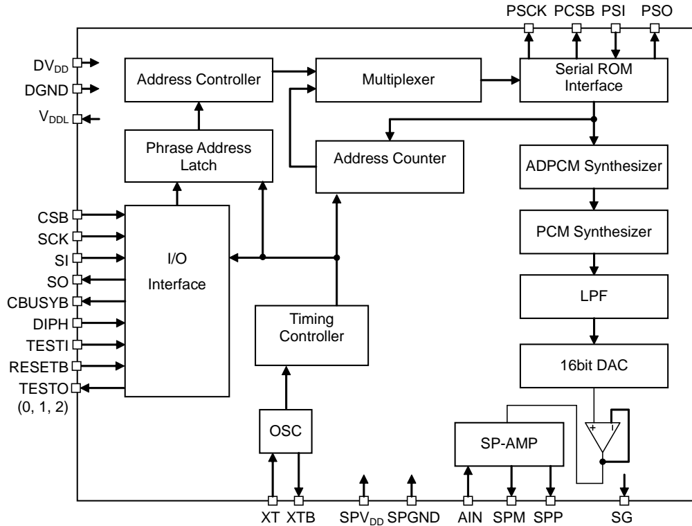
■ ブロック図 (ML22420MB: シリアル同期式インタフェース)
