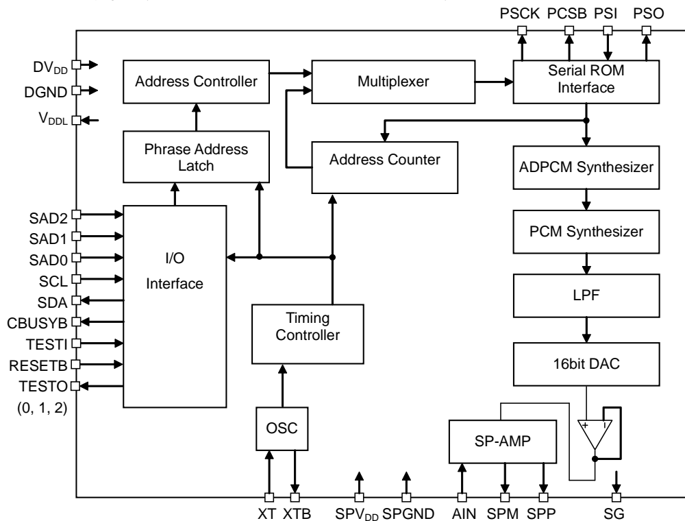
■ ブロック図 (ML22460MB: I2Cインタフェース)
