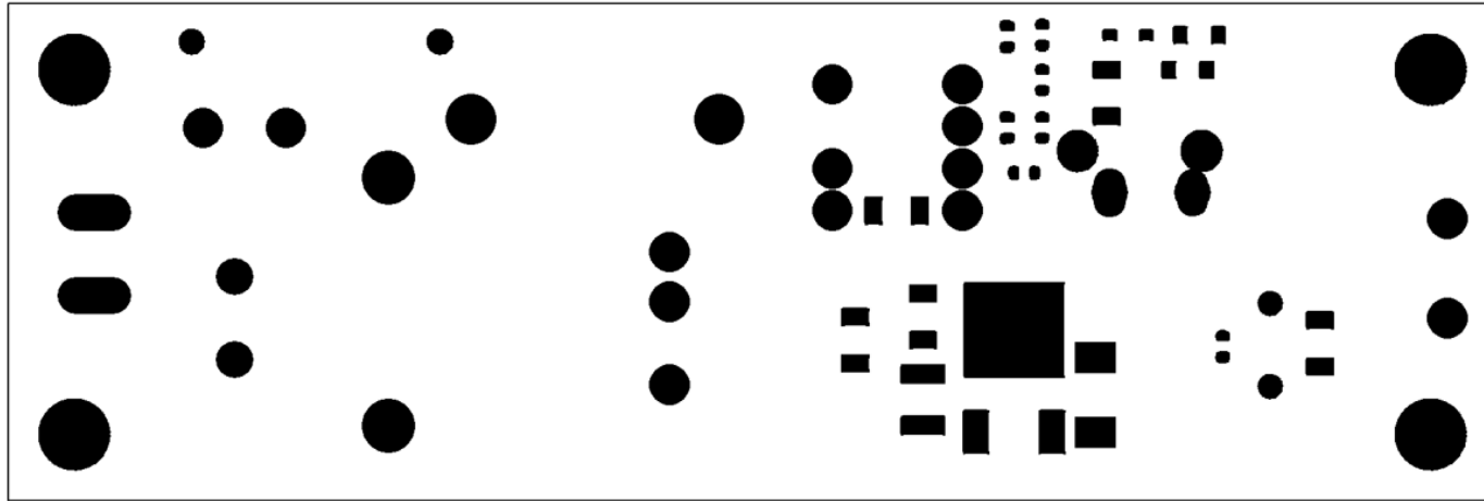
Bottom_Mask
