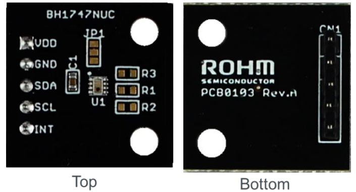
Figure 7. 基板の写真
